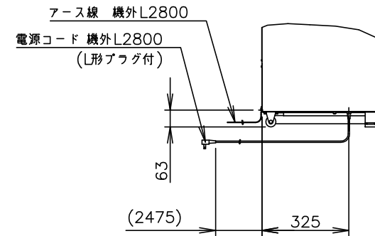
A矢视图 (1/20)
