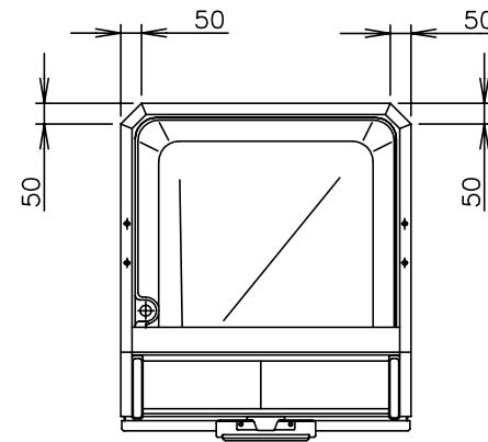
ストッカ上面図
